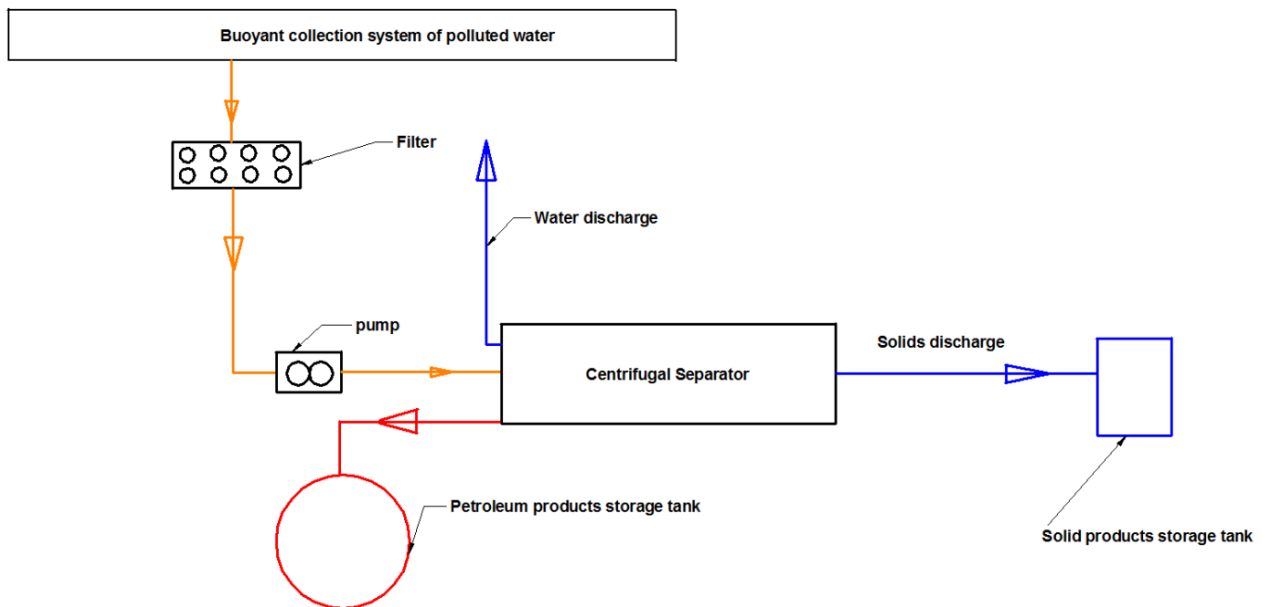
Schema generală pentru sistemul de separare a deșeurilor petroliere
