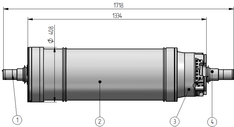
Separator centrifugal-dimensiuni de gabarit
